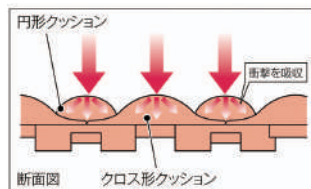
衝撃を吸収する、独自のクッション構造
